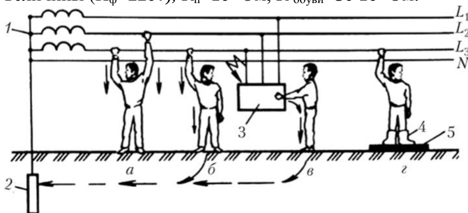
Рис. Схемы включения человека в электрическую цепь
