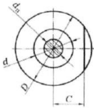
Рисунок 2 - Деталь на оправке
