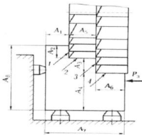
Рисунок 1 – Фрезерование
