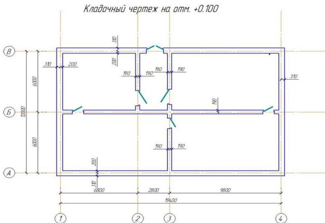
Рисунок 1 – Кладочный чертеж
